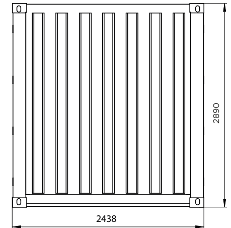
ARRIÈRE
